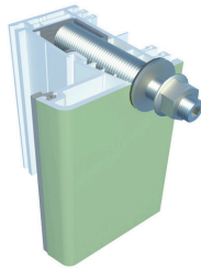
Fix Max® Gewindeanker BS100 für Kunststoff
